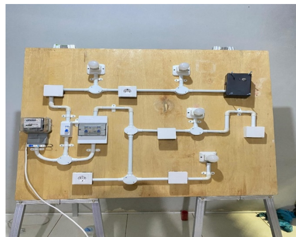
Gambar 1. Desain perancangan alat
